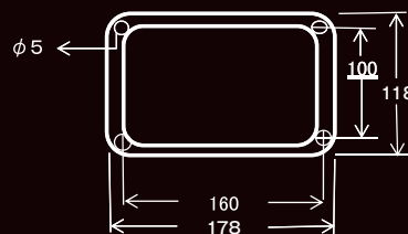
KO灯 開口部寸法〈埋め込み設置の場合〉
