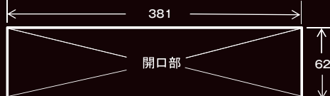
KO灯-S 開口部寸法〈埋め込み設置の場合〉
